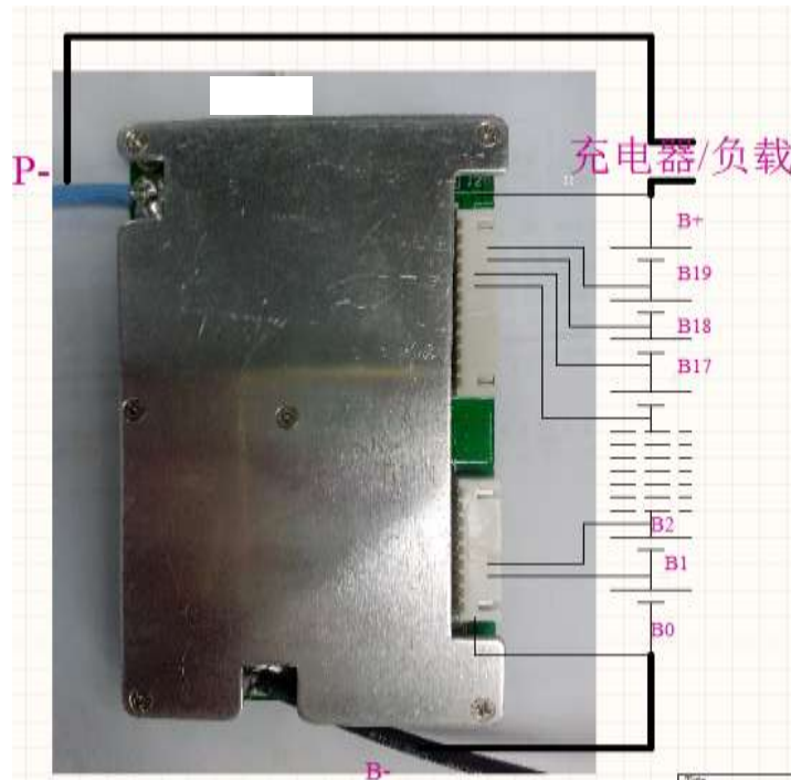
图1. 保护板连接示意图 Figure1 Diagram connection of PC
